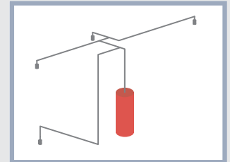
Système d'extinction MX 200 avec un réseau de tuyauteries asymétrique
